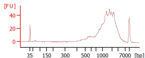
SCN_RGDMH cDNA
