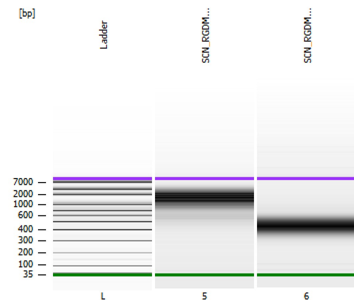
SCN_RGDMH cDNA
