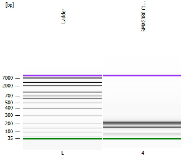
BMAG080 (1:15)
