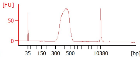
N1015P_N1007Ppippin 325-600bp 4/16 (1:2)
