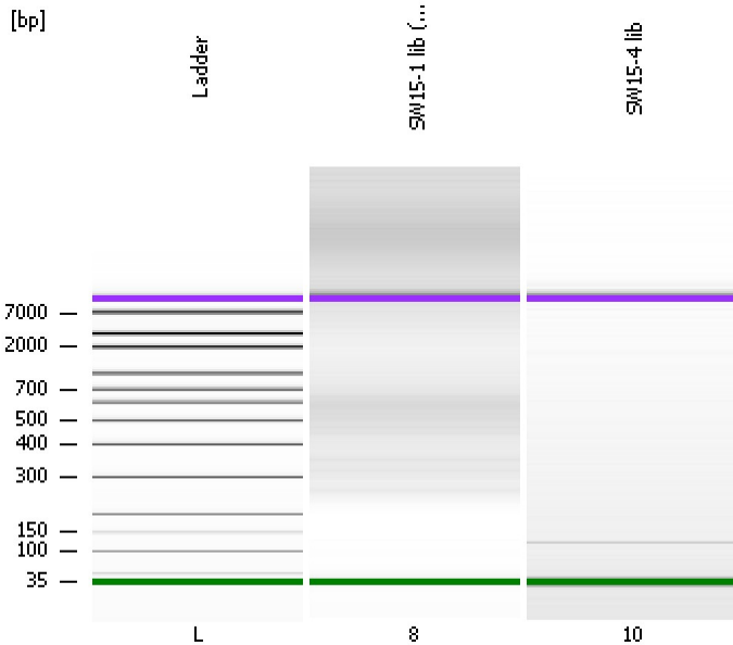
SW15-1 lib (1:20)
