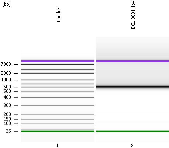
DCL 0001 1:4
