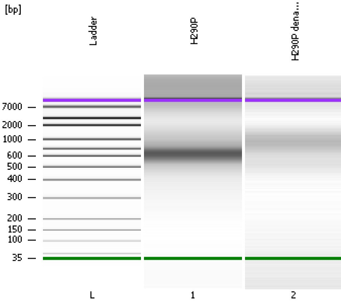
H290P
