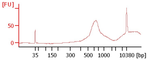
H290P
