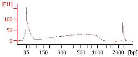
LHC Soni 1:10
