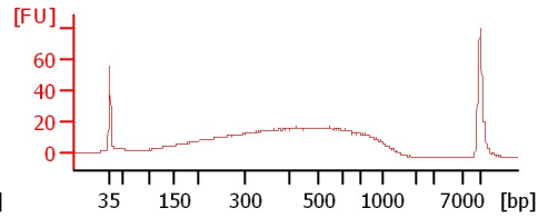
Mickey Soni 1:10
